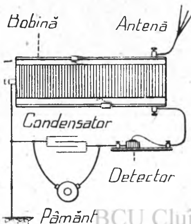
Post radiofonic elementar
