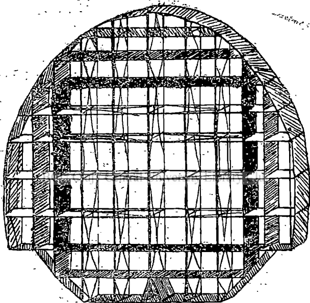
Fig. 12. — Tătură perspectivă schematică prin dirijabilul „Vaugean-Gargiulo”.
