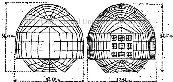
Fig. 13. — Vederea celor două capete a dirijabilului „A-V-3”.
