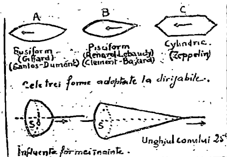
Fig. 6. — Dacă vârful este de formă hemisferică, rezistența aerului la viteza de 10 ser. va fi de 25 kgr., dacă e conic nu va fi decât de 9 kgr.
