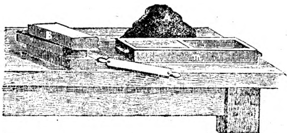
Fig. 5.—Ce trebuie pentru facerea cărămizilor. (A) e lutul muiat cu apă; (B) e forma; (C) e cu ce se rade lutul în formă, iar (D) e cărămida bună.
