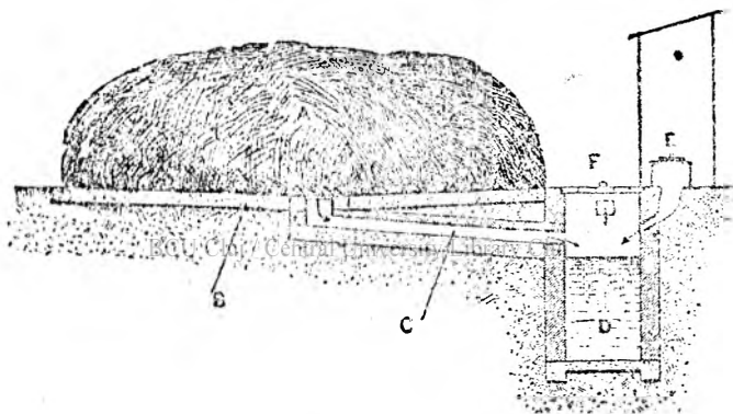
Fig. 2. — Cum e făcut aiurea locul de strâns gunoiul. Aceasta se face căptușă (A) pe podișca (B), aplecată spre mijloc, de unde pleacă o țevile (C), prin care curg zămurile spre vasul din groapă (D). Tot aici se scurg și necurătențiile latrinei.
