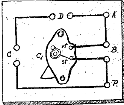
Fig. Nr. 2. Schema de conexiuni.
