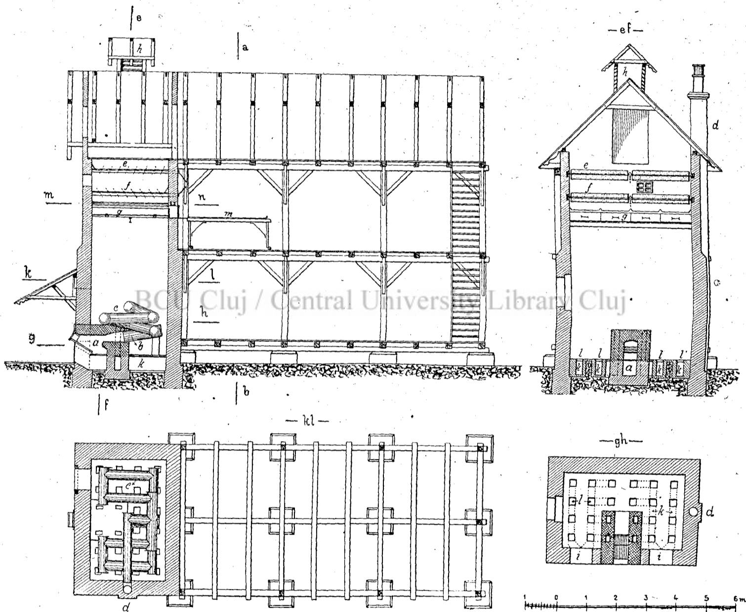
Csehországi (Linhart rendszerű) fűtött komlószárító a kolozsvári gazdasági akadémia telepén. (a. fűtő, b. kazán, c. melegítő-csövek, e., f., g. szárító-rámák, h. szellőző kúrtó.)
