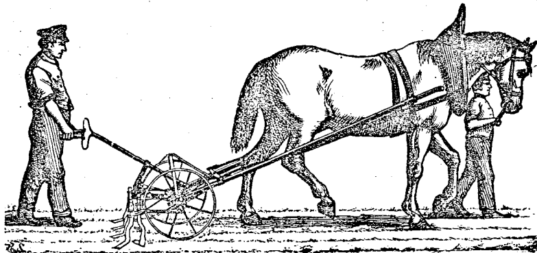
Az egyszerű kapológép. Súlya 4 sor répához való három szerelvénnyel kb. 16 kg.
