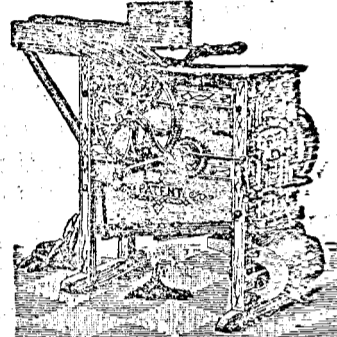
5. Mașină de sfărîmat cunruz! Să afiă cu vînturătoar și fără vînturătoare.
