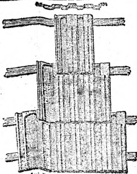
Țigla lui Bohn, patentată Nr. 253, sigură, tescută, dublă și cu supracoperiș.
