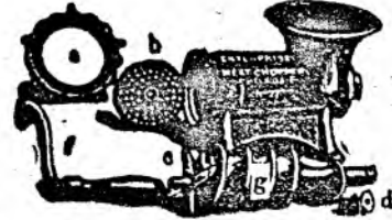
Partile constitutive dela mașina de tocat carne. a) Inel de capac, b) Disc găurit, c) Cuțit, d) Ș rof dela întorcător, e) Întorcător, f) Melciul, g) Taiș. — Fiecare să capătă separat. —
