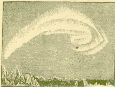
Curioasă formă de auroră polară observată în Laponia; a durat toată noaptea
