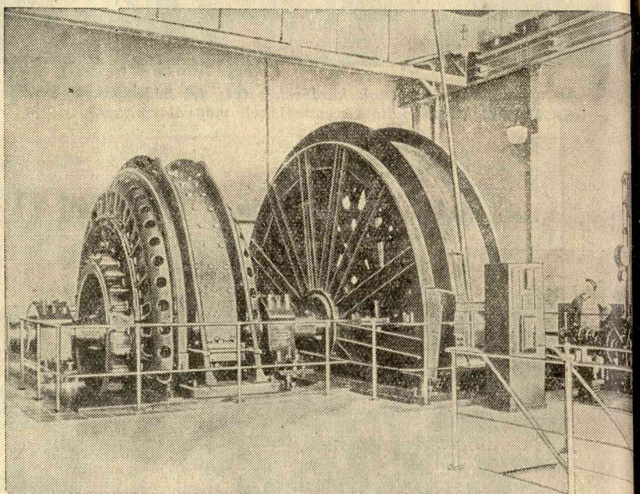
A VILÁG LEGNAGYOBB VILLANYGÉPE. Ez a gépezet a világ legnagyobb villany-húzó gépe, mert naponta 140.000 mázsa széntet tud 1050 méter mélységből felvontatni. Német A. E. G. gyártmány.
