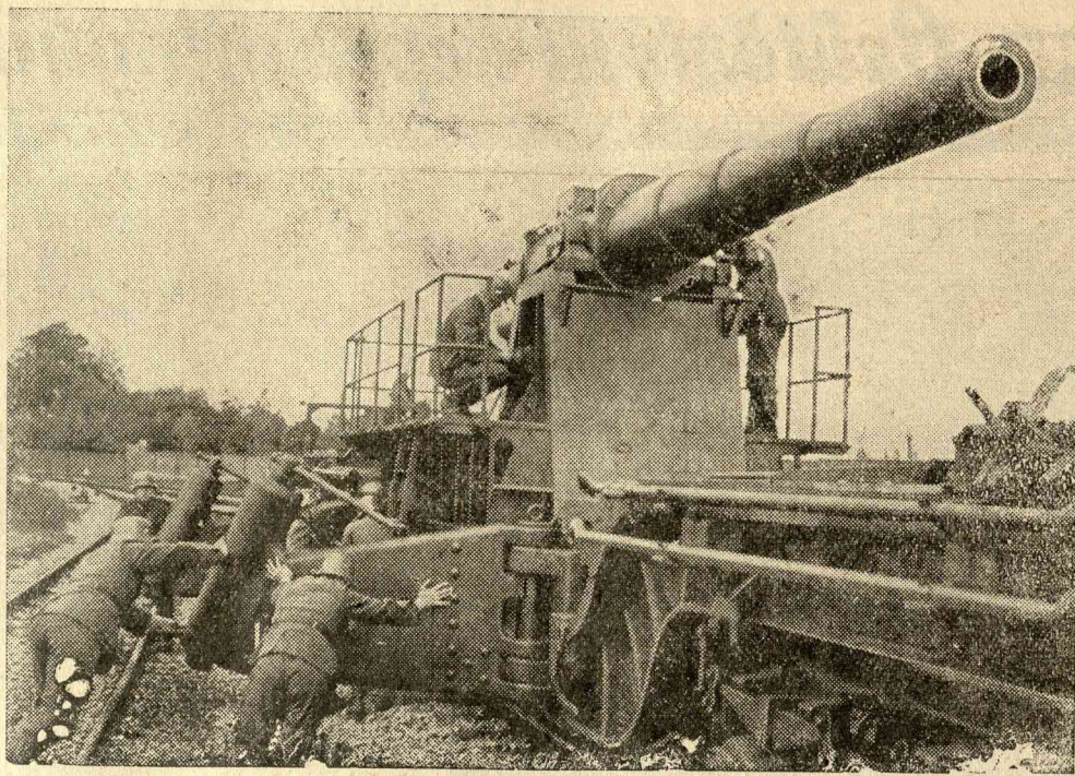
ÓRIÁSI VASUTÁGYU. Képünkön a német hadsereg egyik vasuti ágyuóriását mutatjuk be gyakorlat közben. A gép oldaláról kiálló nagy vaskapcsokat, amelyek arra szolgálnak, hogy az ágyut elsütéskor a talajhoz rögzítsék, a lövés után betolják a számukra elkészített mélyedésbe.
