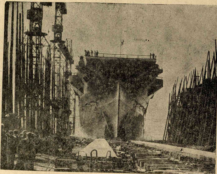
VIZREBOCSÁTIJÁK ANGLIA LEGNAGYOBB REPÜLŐGÉP-ANYA-HAJÓJÁT. A Vickers-Armstrong hajógyár a napokban bocsátotta vízre Anglia legnagyobb repülő gép-anyahajóját, amely 70 repülőgépet vihet magával.
