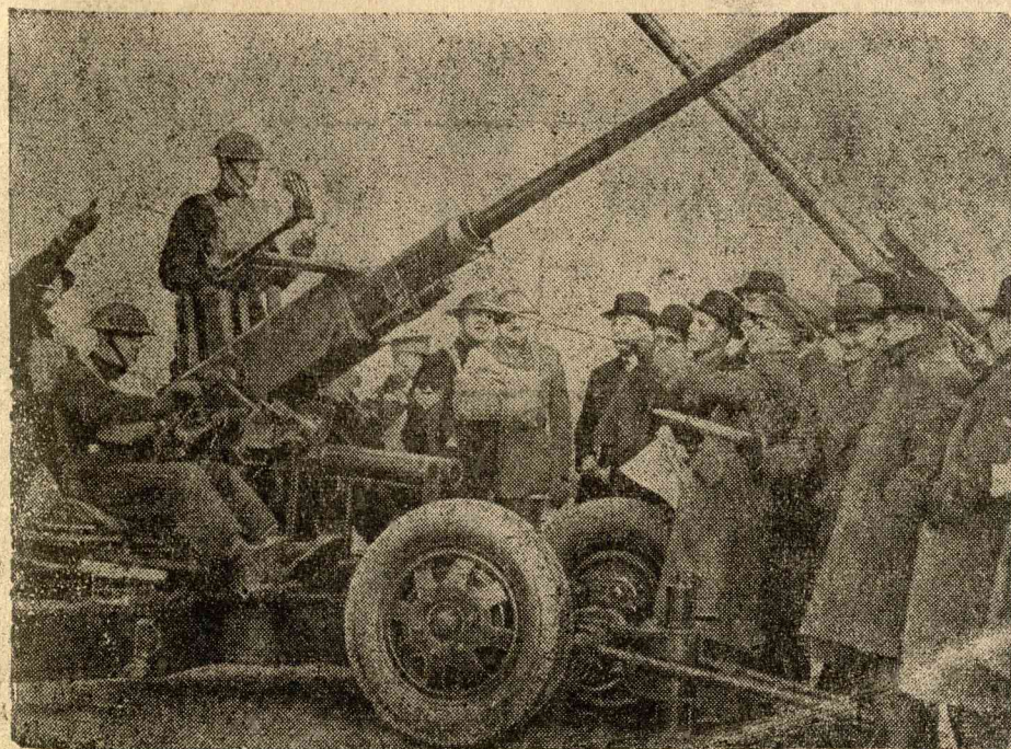
AZ ÚJ ALDERSHOTI LÉGELHÁRÍTÓ ÁGYU. Ez az ágyu percenként 120 lövést tud leadni.
