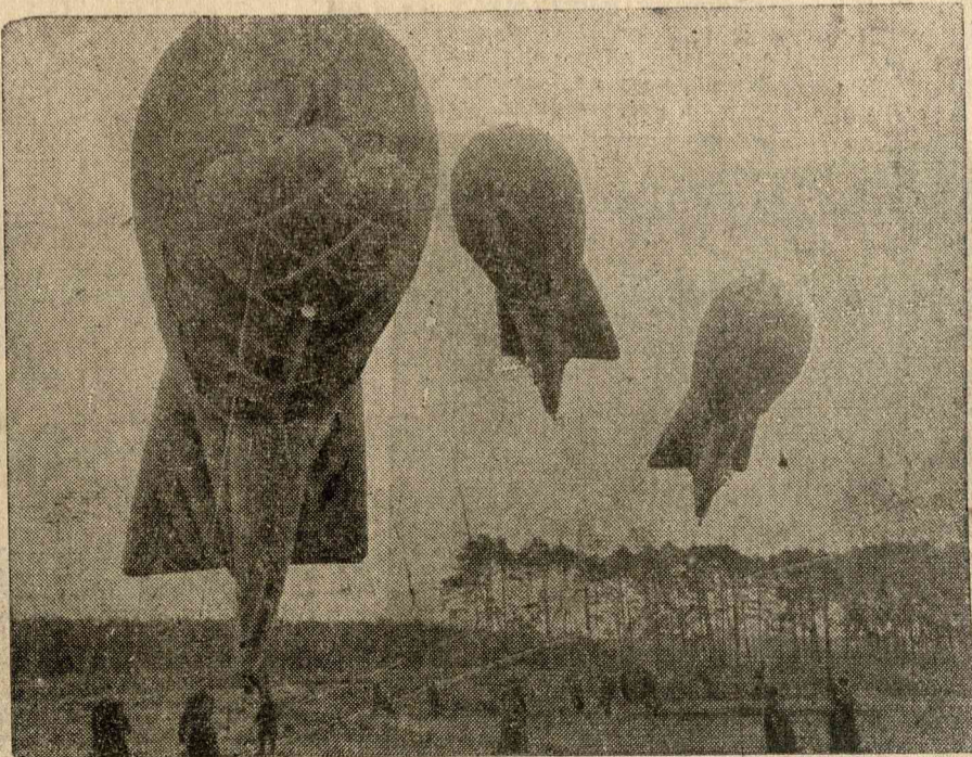
NÉMET LÉGI GYAKORLATOK. Németországban is elsődlegesen megszervezték a légvédelmet, amelynek a kötött ballonok a legjobb eszközök. Ezeket a ballonokat 10.000 méter magasra bocsájtják fel szilárd acélhuzalokon. Ha egy repülőgép a huzalok valamelyikébe ütközik, okvetlen lezuhan.
