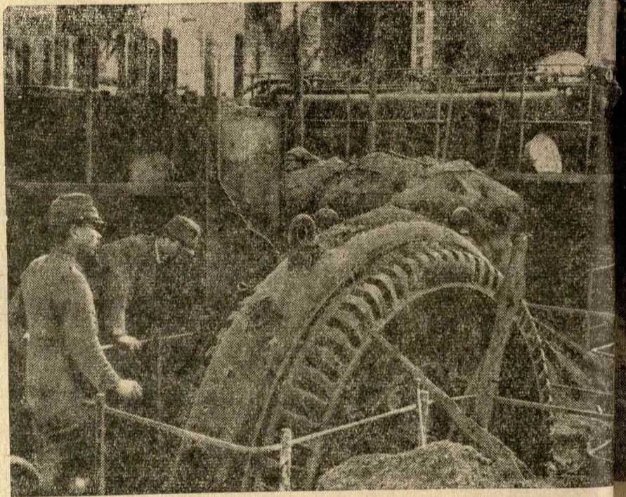
HOMOK A TURBINÁKBAN. A kantoni turbina-művekben a kínaiak mulásuk előtt, hogy használhatatlanná tegyék, homokot hordtak. Ezáltal is az egész ipartelep használhatatlanná tenni.
