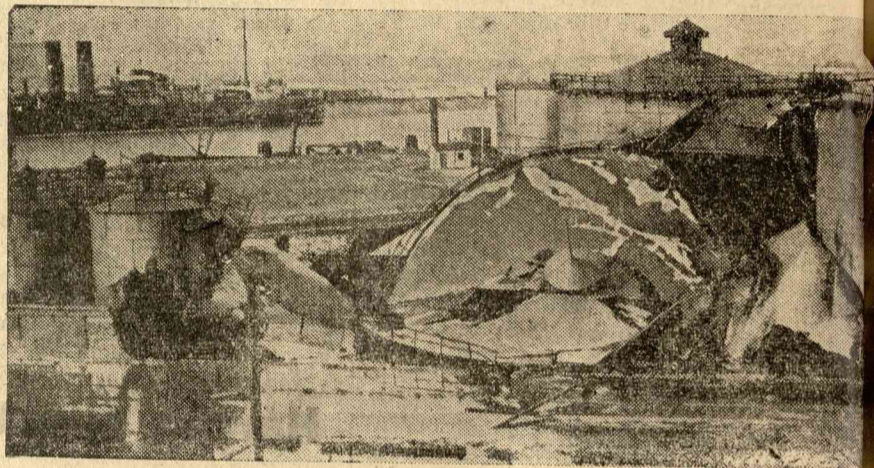
A HIDEG MEGREPESZTETT EGY FOLYÉKONY CUKORRAL TANKOT. Zelbuogeben, Hollandiában nemrég egy folyékony cukorral acéltartályt a nagy hideg megrepszett. A 4000 tonnát kitevő folyékony kárba vesztett.
