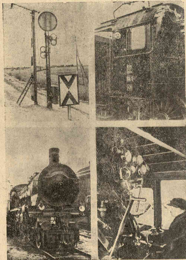
ÖNMÜKÖDŐ MOZDONYFÉK. Fenti képeinken a német vasútvonalakon most alkalmazott önműködő fékszerkezetet mutatjuk be. 1. A fékkampó. 2. A mozdony teteje, ahol egy elektromos hurok áll, amely az állomás előtt felállított fékkampóba ütközik, mielőtt befutna az állomásra. 3. A fékkampó és a hurok összeütközése után nyomban fékez a mozdony. 4. A mozdonyvezető nézi a mozdonyfék működését.
