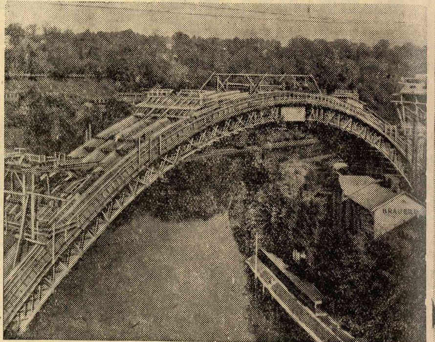
EURÓPA LEGNAGYOBB EGYIVES HIDJA. Bernben most építik meg Európa legnagyobb egyíves hidját, amely, mint a ták be a képünkön látható, valóban imponáló méretű.
