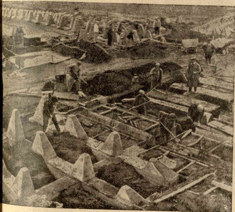
NYUGATI HATÁRERŐDITMÉNYEK. A képünkön látható ak arra szolgálnak, hogy az ellenséges tankok előrehaladását lehetetlenné tegyék.
