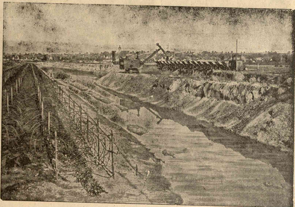
A KELETI NÉMET HATÁROK UJABB MEGERŐSÍTÉSE. Drótaka- dályok és árkok segítségével újabb hatalmas erődtítményeket építenek Né- metország keleti határain.
