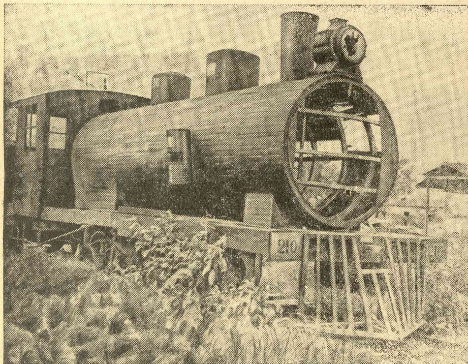
A japán-kinai háborúban a kínaiak egész sor „ál”-mozdonyt szereltek fel Hankeu körül, hogy a japán légihaderő ket megtévedsék.
