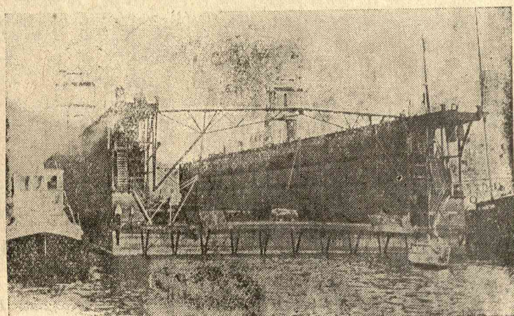
42 NAP TENGERI UT UTÁN megérkezett Constanțăba az a hatalmas uszódokk, amelyet a németországi Lübeckben készítettek és amelyet a romániai kikötőben használnak. Az uszó kikötő 80 millió lejbe került és Constanțăba a Simson és az Albastros vontatóhajók szállították. Az uszó kikötőt lerögzítése pillanatában mutatjuk be.
