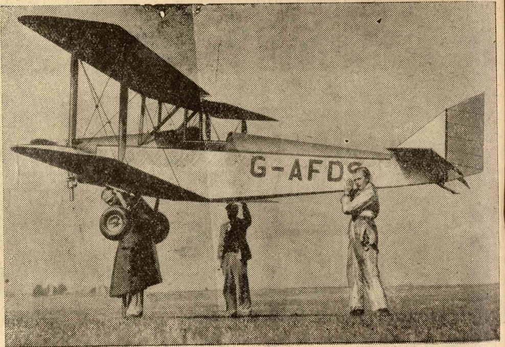
Repülőgép, amelyet két ember elbir a vállán. Ez a repülőgép mindössze 180 kiló súlyu és óránként 9 liter benzint használ és 120 km sebességgel repül.
