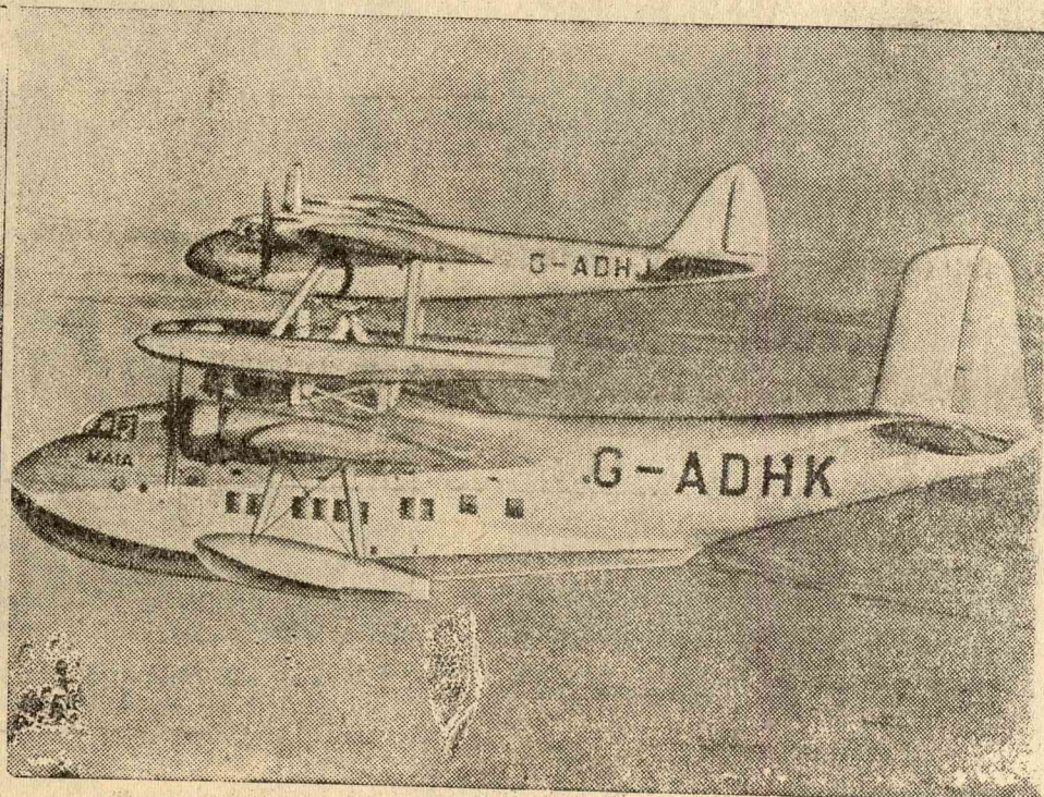
Ikerrepülőgépek repülés közben. Az angliai Rochesterben újfajta, ugynevezett iker-repülőgépekkel kísérleteznek. Együtt emelkednek a magasba, a levegőben azonban a kisebb gép elválik társától és hosszú távolságra indul.
