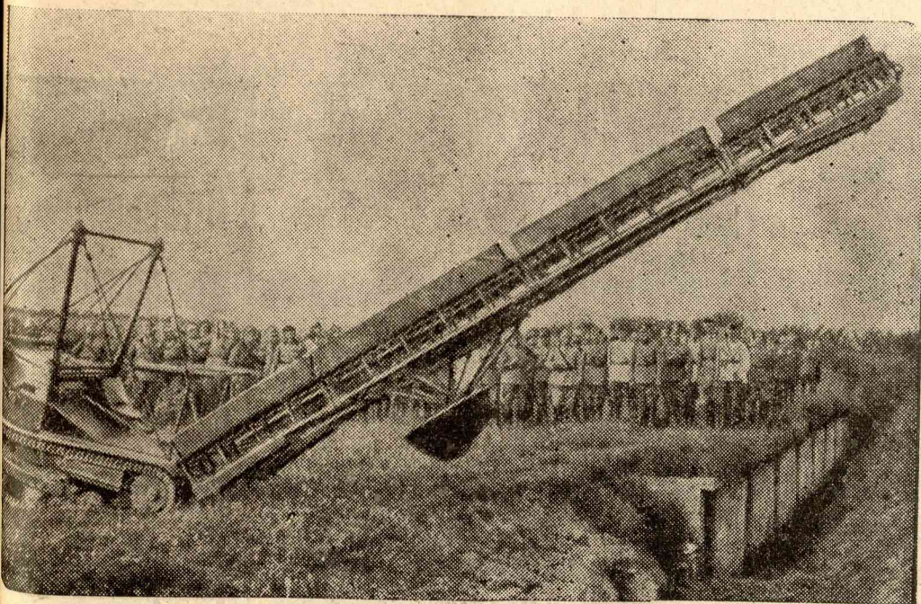
Hidépítő tank. Az olasz hadgyakorlatokon mutatták be a képünkön látható tankot, mely hidakat épít.
