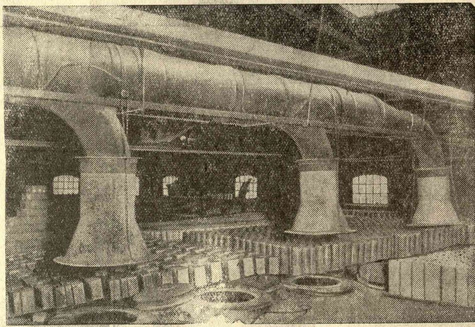
Ujfajta szárító készülék. Németország a négyéves terv sikere érdekében minden energiát leteljesebb mértékben kihasználni igyekszik. Ez a berendezés egy porcellángyáré, melynek kazánjaiból a meleget nem engedik a kéményen át távozni, hanem bevezetik egy szárító terembe és ott felhasználják.
