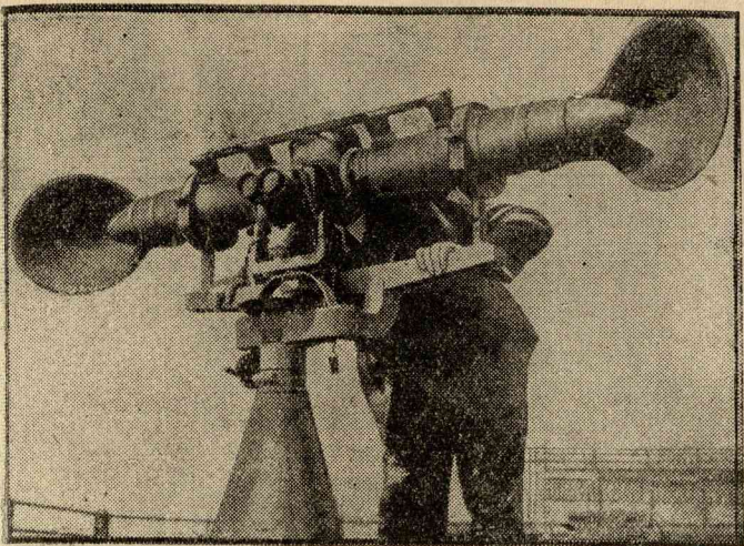
Az elektromos fül. Ezen elektromos szerkezet segítségével több kilométer távolságról meg lehet hallani minden zajt. Különösen a légvédelmi ütegek számára rendkívül fontos ennek alkalmazása.
