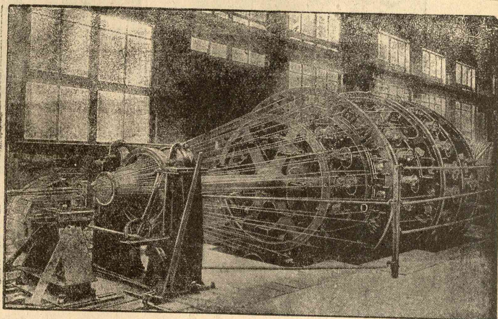
A kábelsodró gépek működés közben. Óriási gépek sodorják össze és foglalják közös burkolatba a hatalmas súlyú és vastagságú kábeleket, melyeket a tengerentúli beszélgetések lehetővé tételére raknak le.
