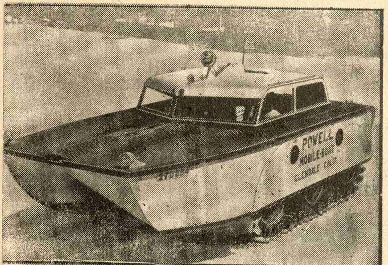
Autó, mely csónak is egyszerre. George Powell angol mérnök készítette a fenti csónakot, melynek az a sajátossága, hogy szárazföldön is igen nagy sebességet tud elérni
