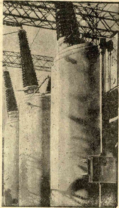
Az erő megtestestítése. Három óriási kapcsoló, melyek a világ legerősebb áramának vezetői. A drótokon ugyanis 280 ezer Voltot vezetnek 1200 Ampérellel.
