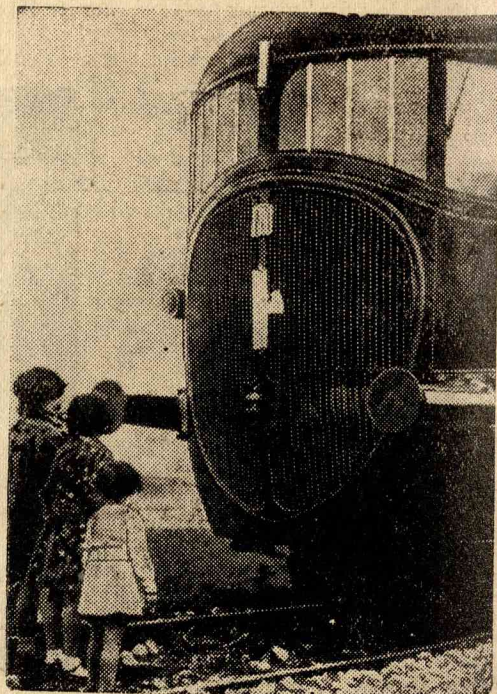
Az áramvonalas mozdony hűtővel. A milánó-nápolyi útvonalon fog közlekedni. Érdekessége, hogy a mozdonynak gépkocsiszerű hűtője van.
