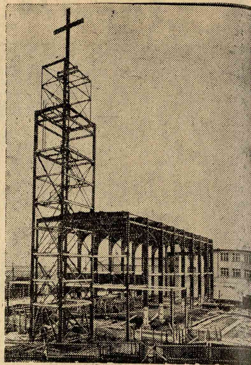
Az első acélvázú templom Csehszlovákiában. Mährisch-Ostriban, amely Csehszlovákiához tartozik, megkezdtek az első acélvázú templom építését. A templom 37 méter hosszú, 12 méter széles.
