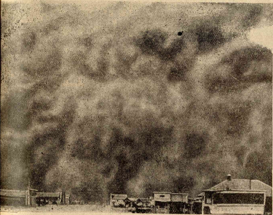
A Kansas-i számun. Kansasban Északamerikában a Szahara sivatához hasonló óriási homokvihar tombolt. Ezen viharfelhőket mutatjuk, amint igen nagy gyorsasággal közelednek egy farm felé.
