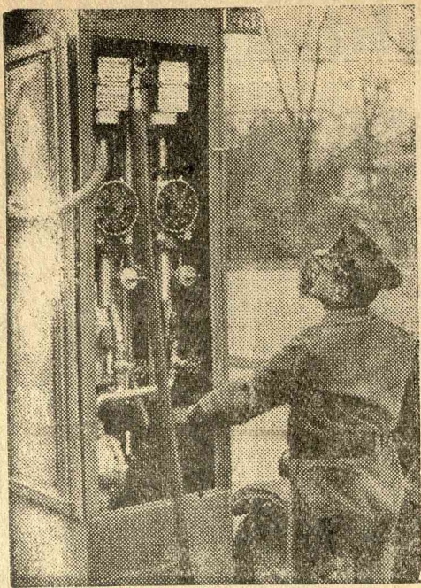
Villamos benzinpumpa. Berlinben most állították fel a legmodernebb villanyerőre berendezett benzinpumpát, amely percenként 60 liter mennyiséget tud az autókba átömlesztetni.
