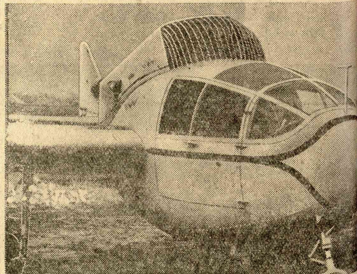
A „repülő ló tojás.” Az amerikai Hayden Campbell a képünkön látható különös alaku repülőgéppel 190 kilométeres sebességet ért el óránként.
