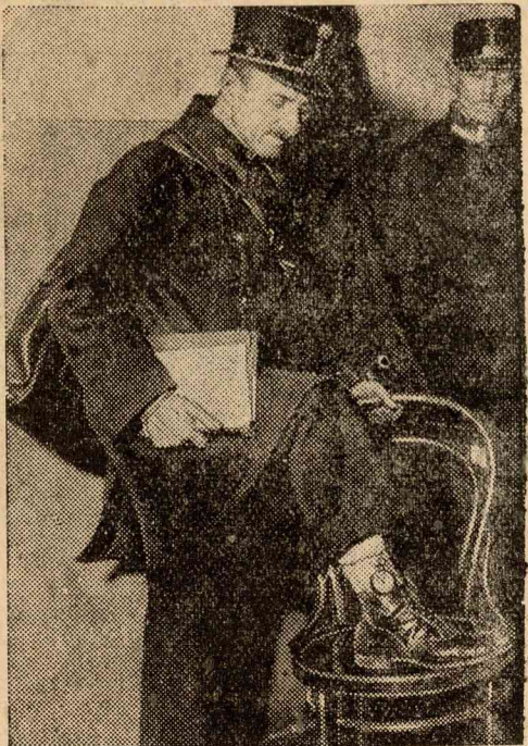
A budapesti állami postahivatal igazgatósága lépésmérővel látta el a postásokat. Amint látjuk: a szerkezet a levélhordó lábára van csatolva s így akarják pontosan megállapítani, hány kilométert tesz meg egy postás.
