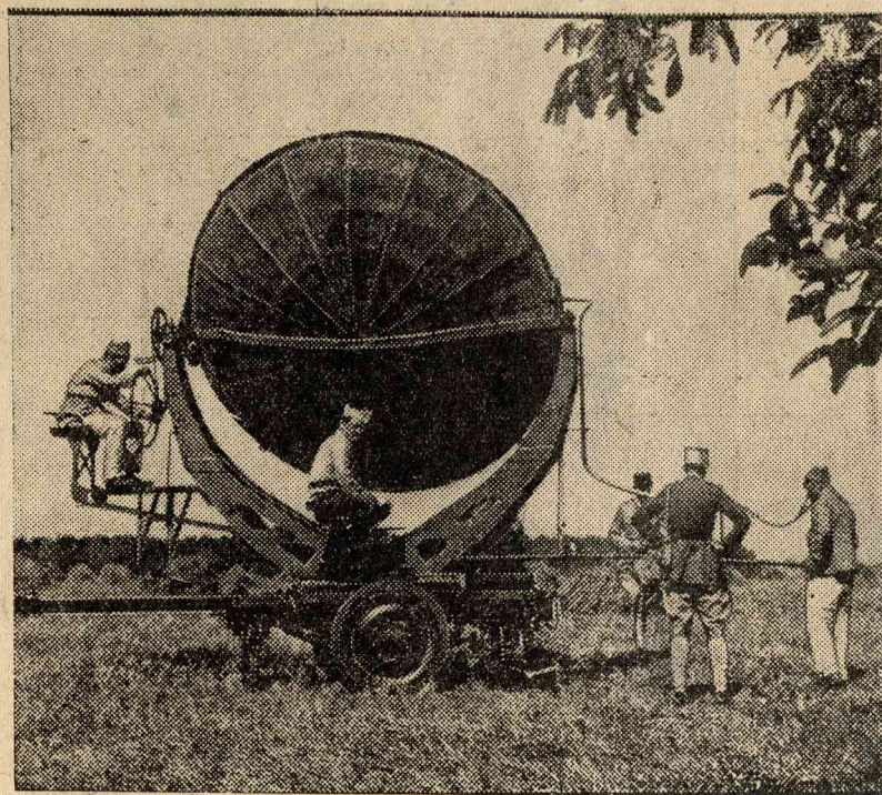
A francia légi hadgyakorlatokról. Képünk azt a készüléket ábrázolja, mely a közeledő repülőgépek motorok zaját igen nagy távolságról jelzi.
