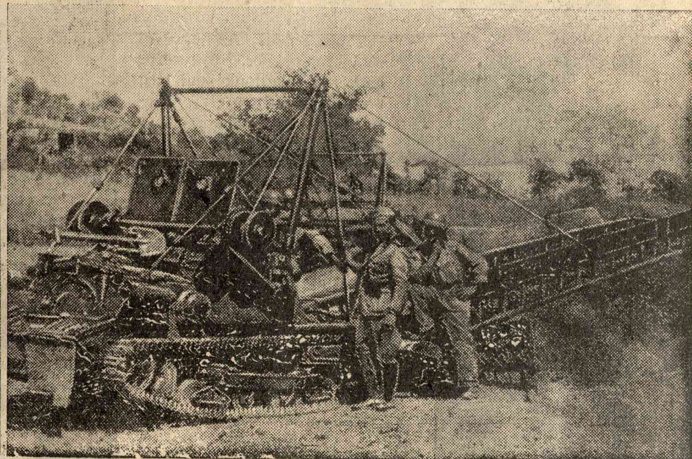
Harciközi saját hidakkal. Az Olaszországban lefolyt hadgyakorlatokon új hadieszközöket vezettek be, többek között azokat a tankokat is, amelyek alkalmasak lehetnek arra, hogy önmagukból tűzoltó-létraszertűen hidakat bocsássanak ki, melyeknek segítségével 5—10 méteres akadályokat áttudják hidalni.
