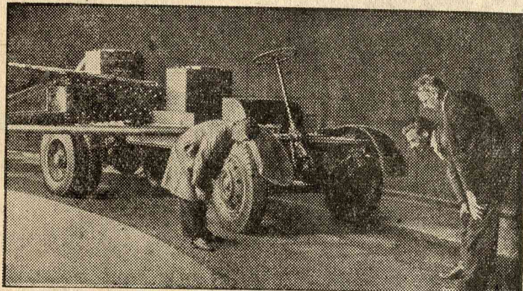
ÚJ KÉSZÜLÉK AZ UTAK TEHERBIRÓ KÉPESSÉGÉNEK MEGÁLLAPÍTÁSÁRA
