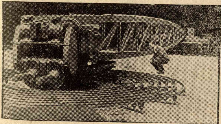
ÚJ KÉSZÜLÉK AZ UTAK TEHERBIRÓ KÉPESSÉGÉNEK MEGÁLLAPÍTÁSÁRA
