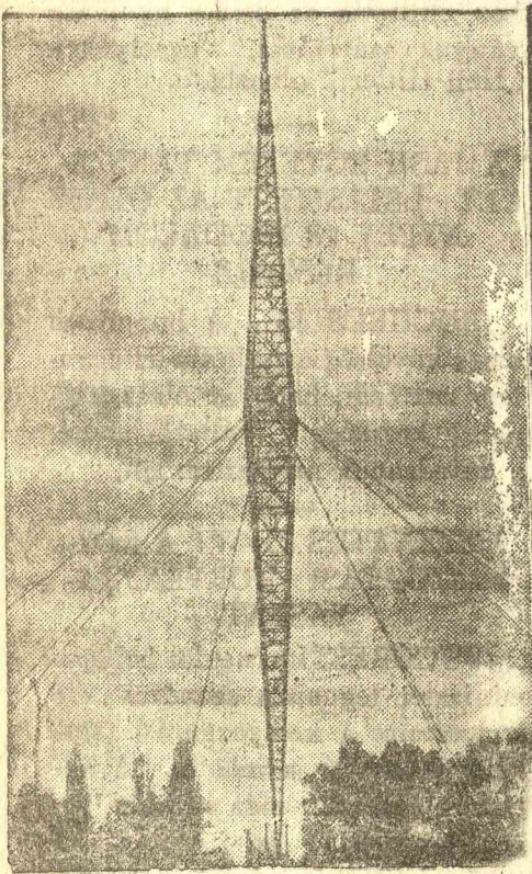
A LEGMAGASABB ANTENNA TORNIA, a 314 méter magas új budapesti nagydó, amely a párisi Eiffeltoronytól 14 méterrel magasabb. Felső végén időjárásjelző műszer van.
