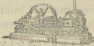
COMPOUND GŐZGÉP
