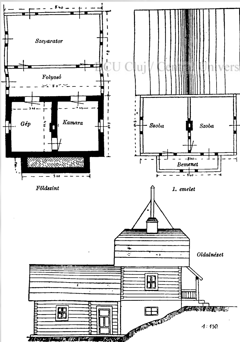
10. ábra. Mencesli tanya és gépház tervrajza.
