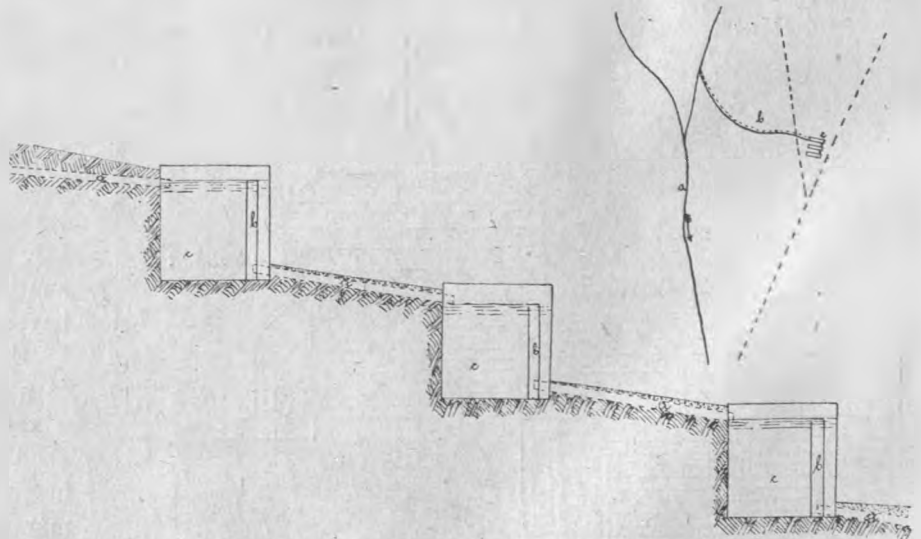
12. ábra. Fent: Földalatti csövek a tervrajza, mellyel a vízet a vályuhoz vezetik. Lent: A vályuk elhelyezése.
