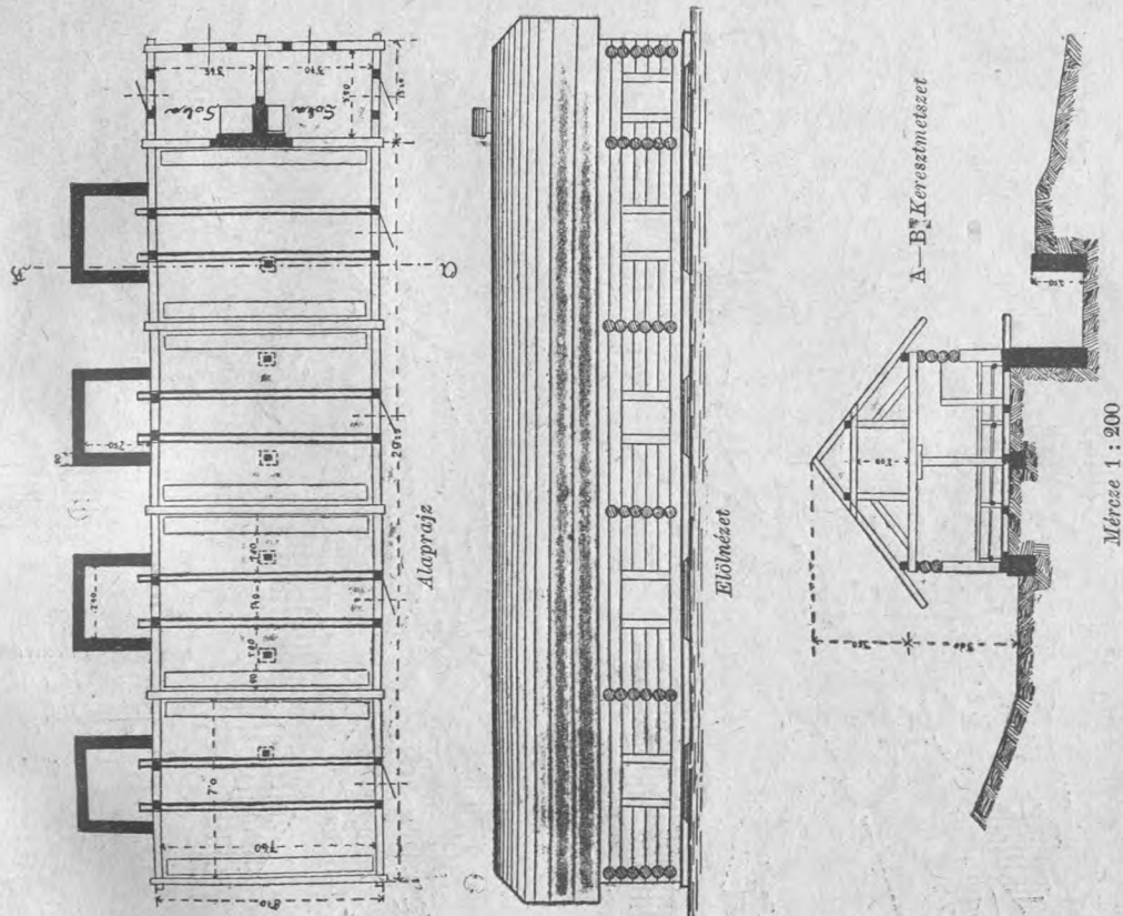
5. ábra. Istálló keresztfekvéstű jásszallal.
