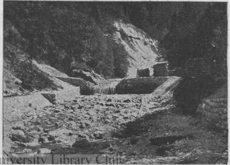
11. kép. Offensee: Kőből épült lépcső.
