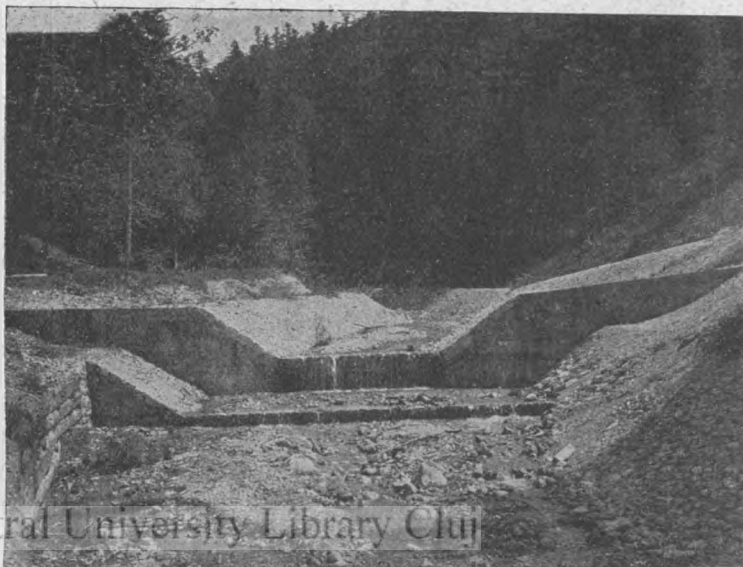
12. kép. Offensee: Beton-lépcső.
