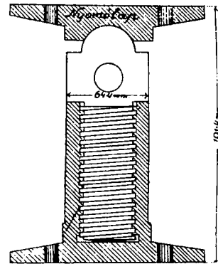
Nyomólap alárajza
