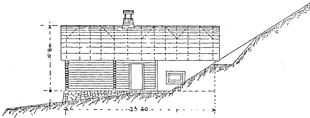
Hossznézet.
