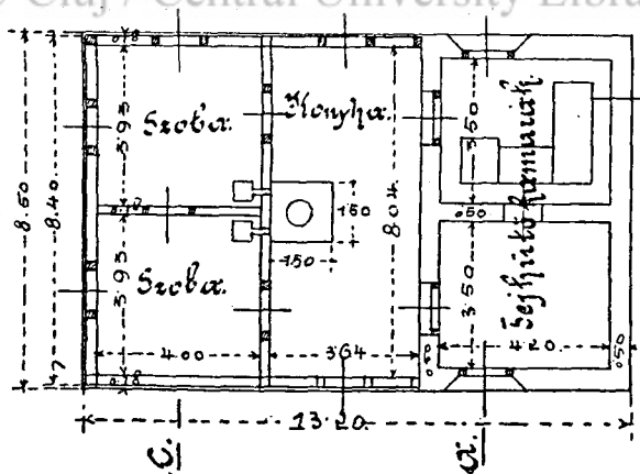
Alaprajz.
