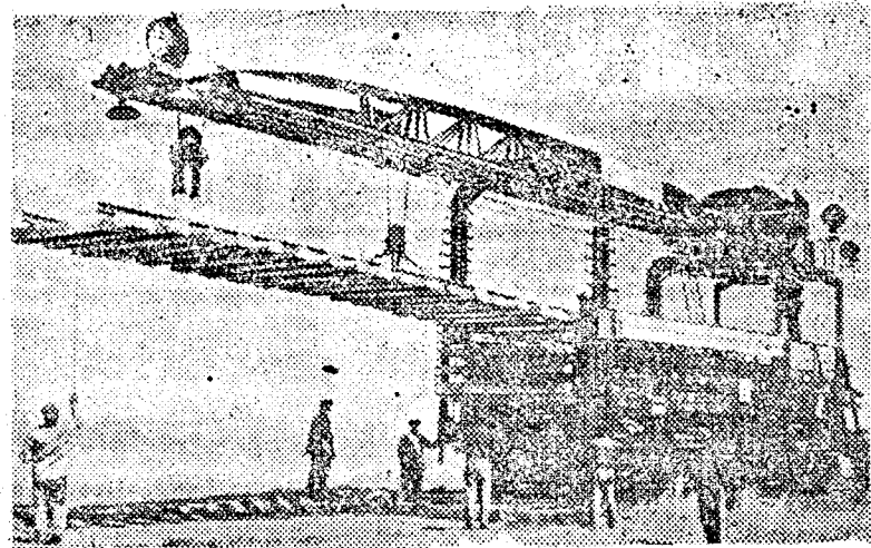
Talpfákra előre felszerelt vágányokat helyez a töltésre és tovább gördül a síneken Pletov mérnök talpmánya. A gép nagymértékben megkönnyíti az ember munkáját és meggyorsítja a vasutépítést.
