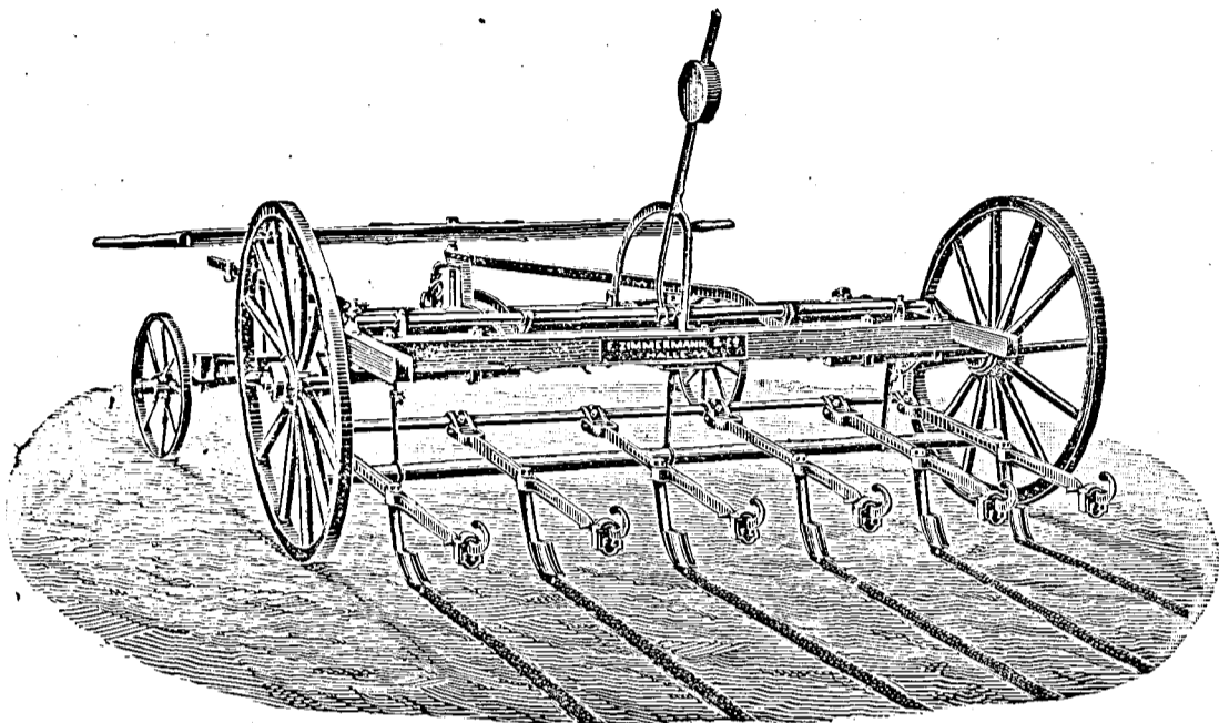
1. ábra. A burgonya kultivátor mint sorhuzó.
