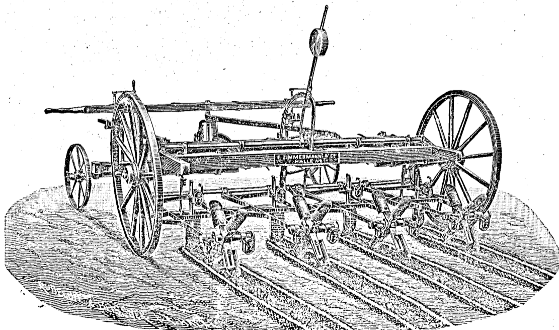
2-ik ábra. A burgonya kultivátor fészekvájóul beállítva.
