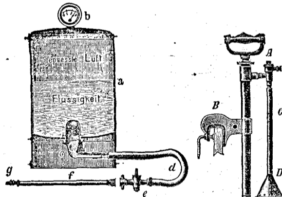
1. ábra. A Mayfarth és társai „Syphonia“ szőlő- és növény-permetezője. 2. ábra. 1. tartány. 2. szivattyú.
