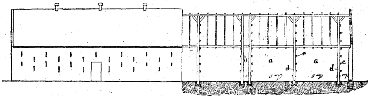
1. ábra. Dohányszárító pajta oldalról és hosszmetsetben.
