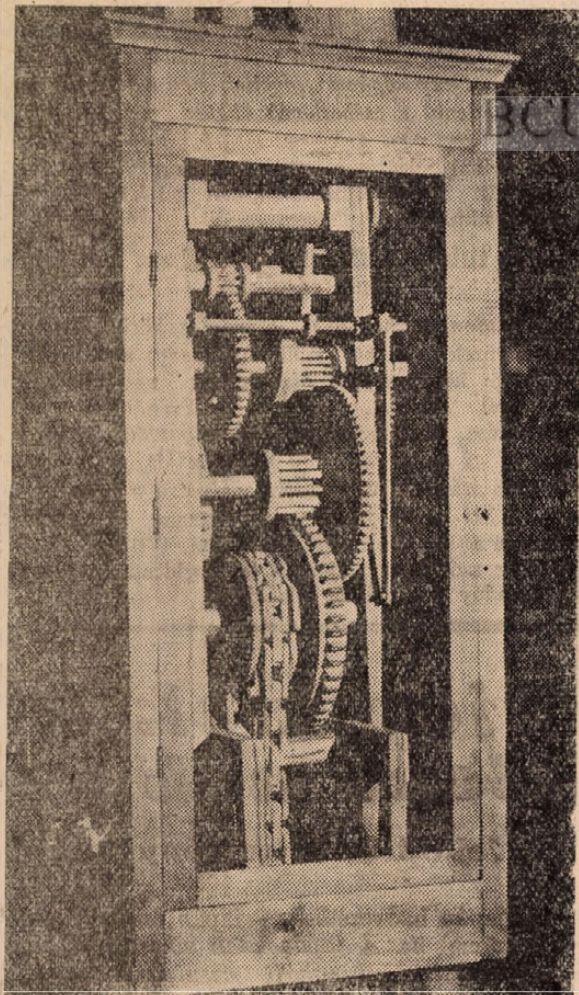
A csodaóra szerkezete (oldalnézet).
