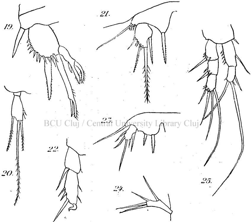
FIG. 19—21. Canthocamptus Georgevitchi . — FIG. 19. Régénération de la seconde paire de pattes ♀. — FIG. 20. Endopodite de la quatrième paire de pattes. — FIG. 21. Patte de la cinquième paire ♂. FIG. 22—25. Moraria Stankovitchi . — FIG. 22. Endopodite de la quatrième paire de pattes ♂. — FIG. 23. Patte de la cinquième paire ♂. — FIG. 24. Branche accessoire de la seconde antenne. — FIG. 25. Patte de la première paire ♀.
