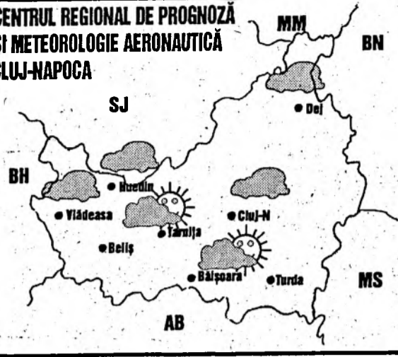
Harta privind starea probabilă a vremii în județul Cluj, valabilă pentru 13.01.1997, în jurul orei 15.
