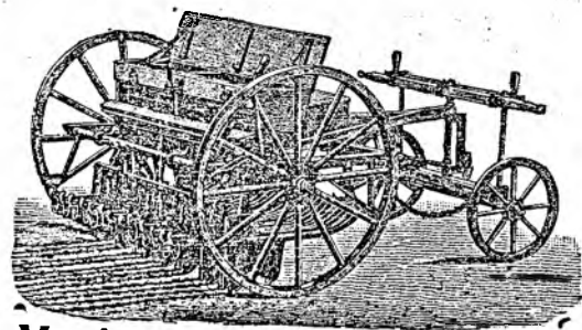
Mașină ușoară de sêmănat „Königs Drill“.
